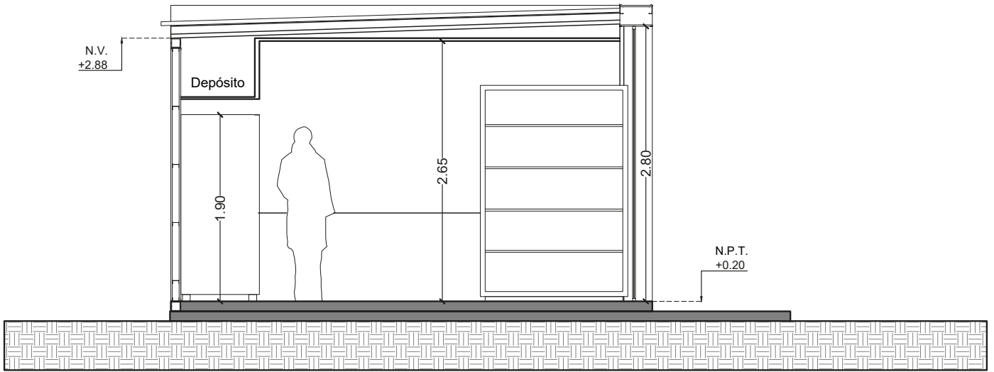
CO CORTE 2-2 ESC.: 1:50
