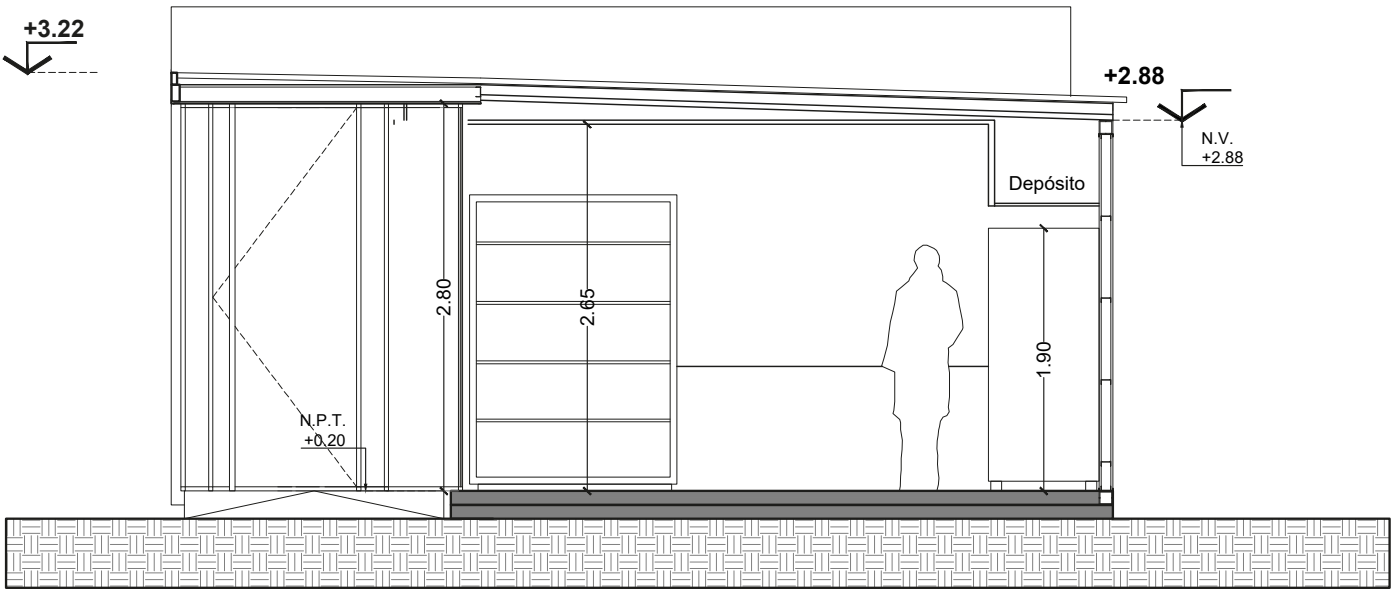
CO CORTE 3-3 ESC.: 1:50
